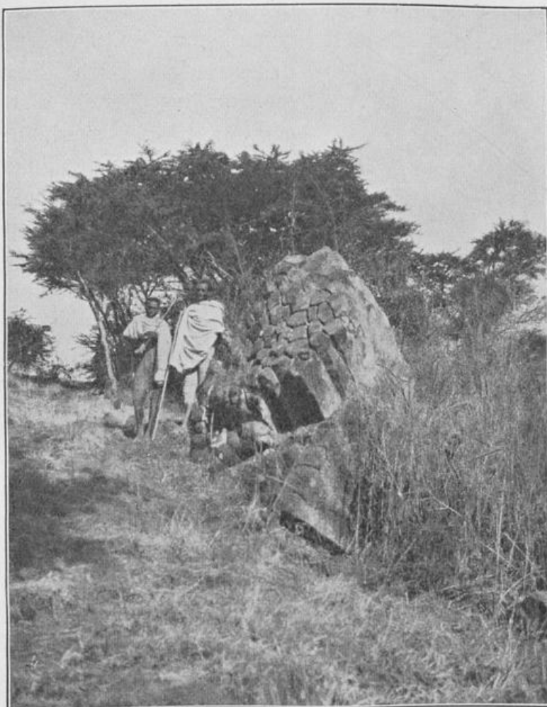
Engbegrenzte Basalteruption, Tigre, unfern von Aksum (Photographie C. Bosch)
