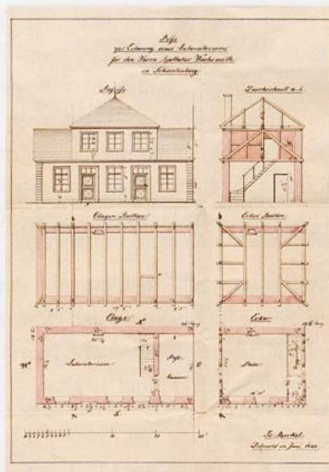
Plan zur Erbauung eines Laboratoriums für den Herrn Apotheker Wachsmuth in Schwalenberg. (Detmold im Juni 1842).
