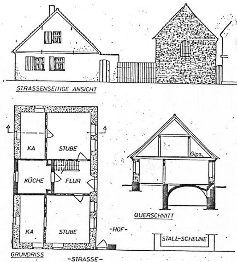
Wohnhaus eines Landarbeiters in Bottmersdorf, Kreis Wanzleben (816/24) Rach 1882, 192
