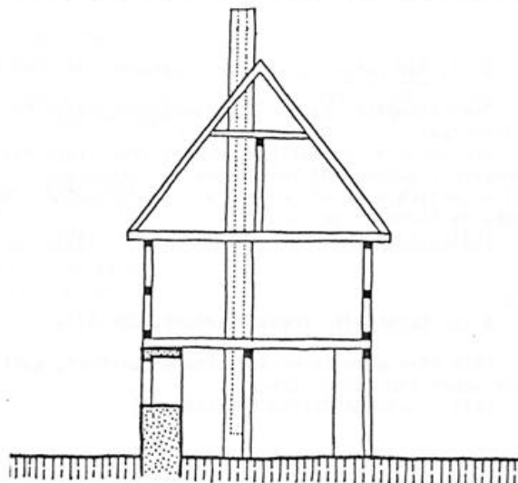
Senkrechter Schnitt o.M. Bernbruch Nr. 37
