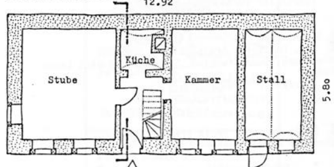
ehemaliges Gärtneranwesen Döben Nr. 27
