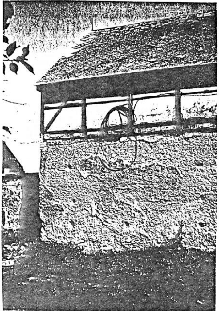
Kaditzsch, Kreis Grimma "Lehmstock". Die Löcher der Traversen der Stampf- schalung wurden bewußt belassen, um die Lehmstampf- wand besser austrocknen zu lassen und um die Räume zu ventilieren. Vom ehemaligen Außenputz sind nur noch Reste erhalten. (Foto : Verfasser)
