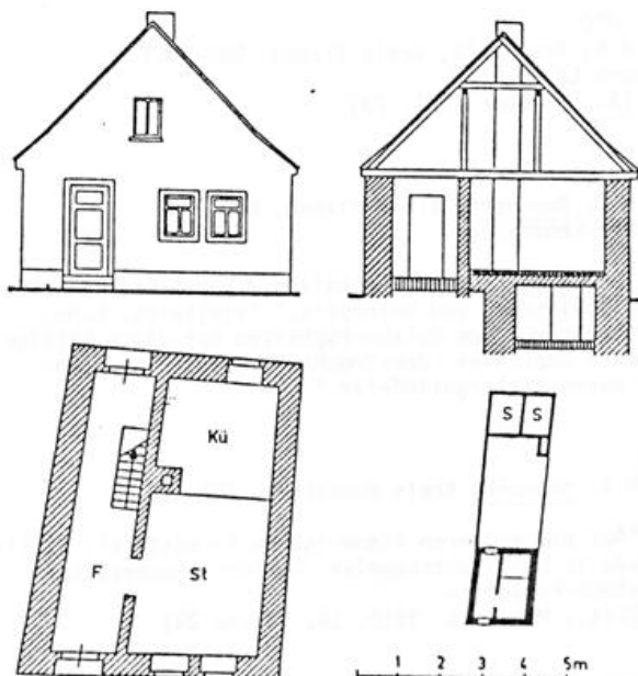
Abb. 36. Gutsarbeiterhaus in Olbersleben, Kr. Stimmerda, von ca. 1800. Lehm Bau. Ansicht, Querschnitt, Grundrisse des Hauses und Anwesens. F Flur, St Stuhenteil, Kü Küchenteil des Wohnraums, S Schweinestall
