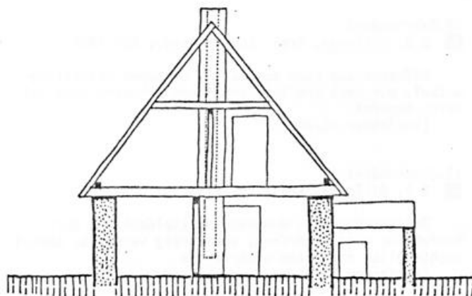
Senkrechter Schnitt o.M. Häuslerhaus Bernbruch Nr.21
