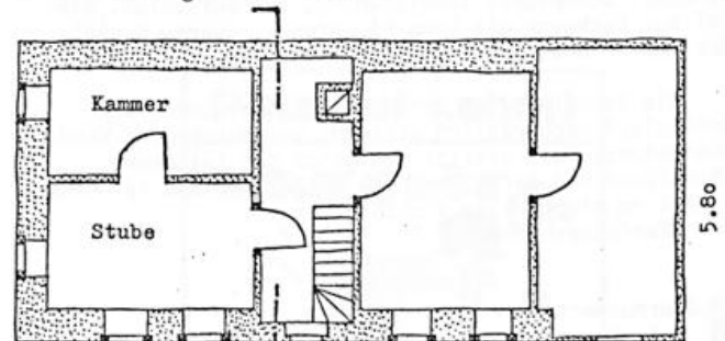
Grundriß Obergeschoß o.M.
