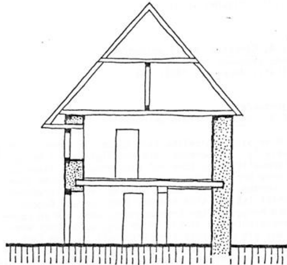
Senkrechter Schnitt o.M. Gärtnieranwesen Döben Nr.27
