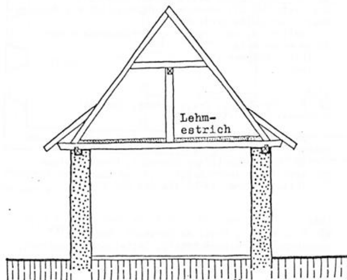
Senkrechter Schnitt o.M. Stall Bernbruch Nr.13
