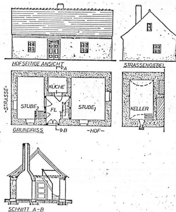
Wohnhaus eines landarmen Dorfbewohners ("Häusler") in Atzendorf, Kreis Staßfurt. Rach 1882, 186
