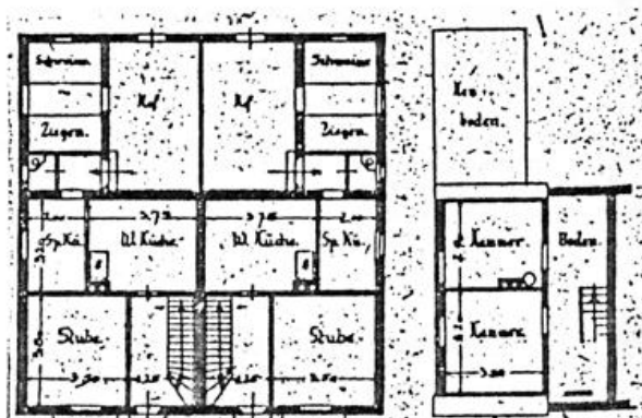
Abb. 14. Erdgeschoß. M. 1:800. Abb. 15. Dach.
