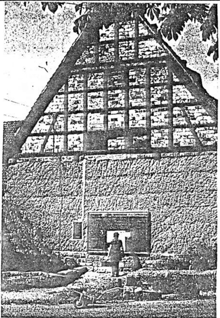
Dothen, Kreis Jena. Scheune mit Umfassungswänden aus Stampflehm. Die Stampfschichten sind noch gut zu erkennen. (Foto : Verfasser)
