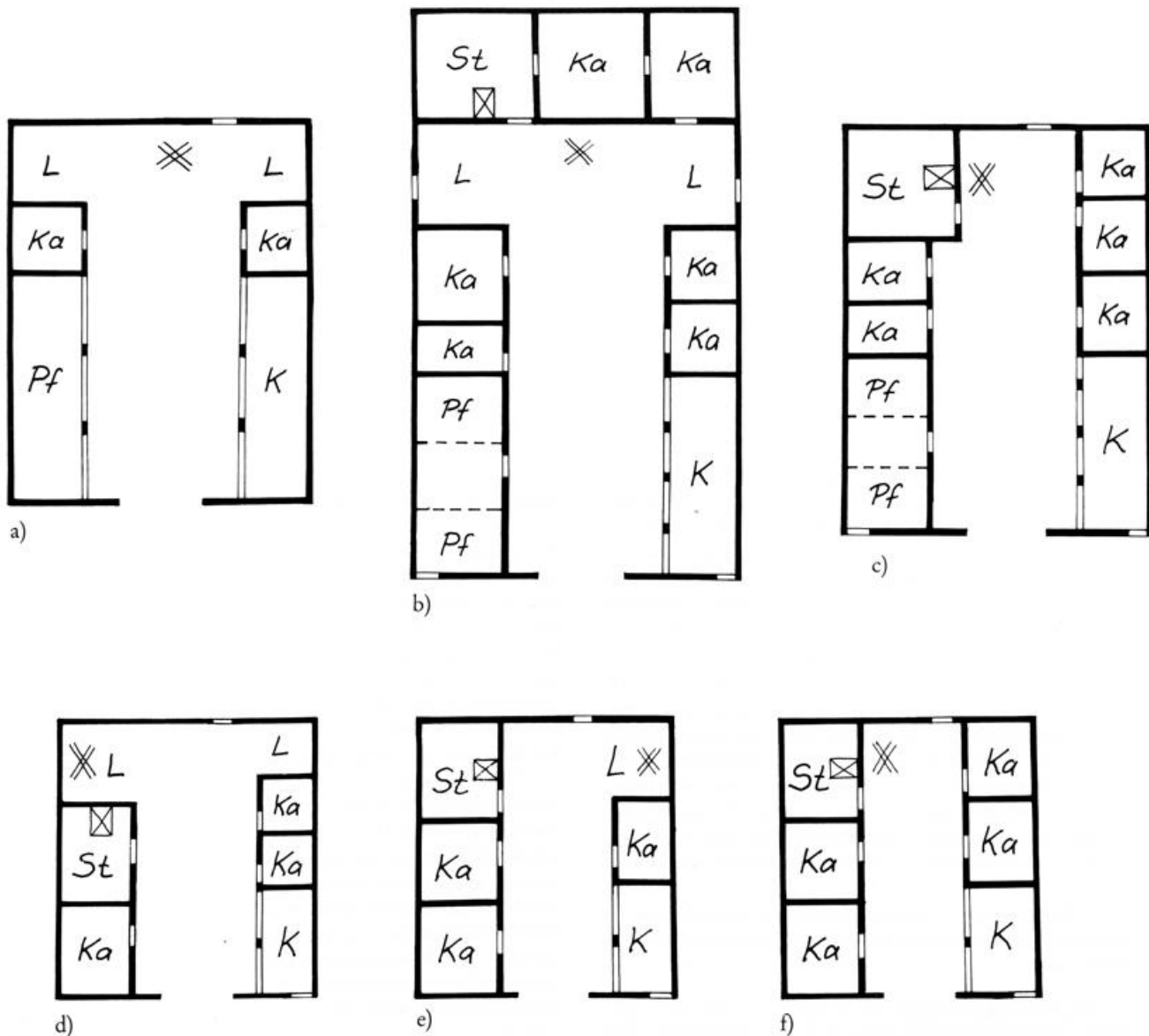
Abb. 10: Obere Reihe: Grundrißformen lippischer Bauernhäuser (schematisch): a) Flettdeelenhaus ohne Kammerfach; b) Flettdeelenhaus mit Kammerfach; c) Durchgangsdeelenhaus mit großer Stube in Ecklage. Untere Reihe: Grundrißformen lippischer Kötterhäuser (schematisch): d) Flettdeelenhaus ohne Kammerfach mit Küchenlucht; e) Durchgangsdeelenhaus mit großer Stube in Ecklage; f) reines Durchgangsdeelenhaus ohne Luchten, Herdstelle am Ende der schmalen Deele. St = Stube, Ka = Kammer, L = Lucht, Pf = Pferdestall, K = Kuhstall.
