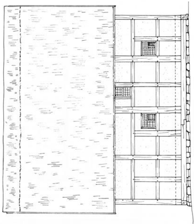
WEST-ANSICHT
