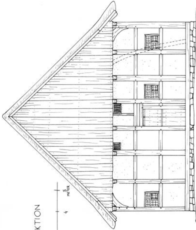
SÜD-ANSICHT
