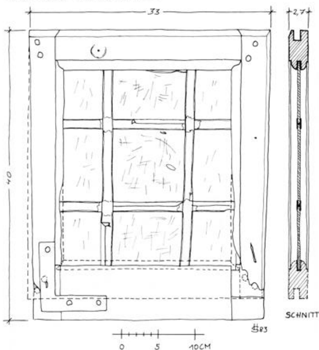
TEIL EINES SCHIEBEFENSTERS MIT BLEISTROSSEN — BEFUND, URSPRÜNGLICHER ZUSTAND GESTRICHELT — Abb. 78.
