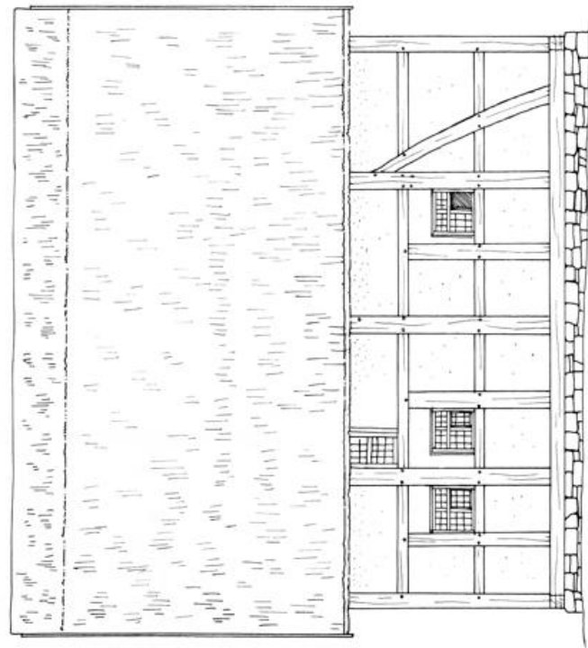
ÖST-ANSICHT
