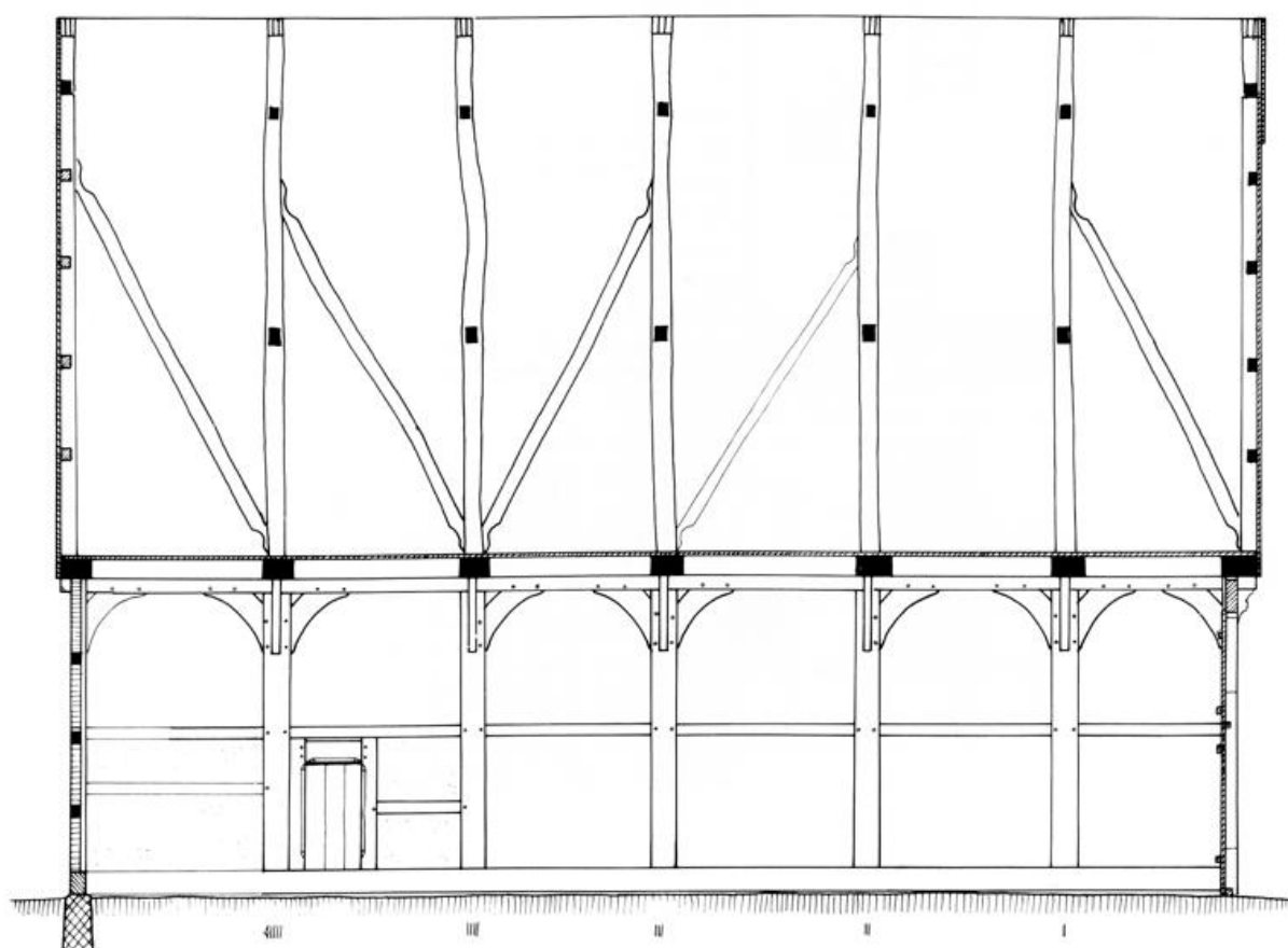
LÄNGENSCHNITT E-F - REKONSTRUKTION -
