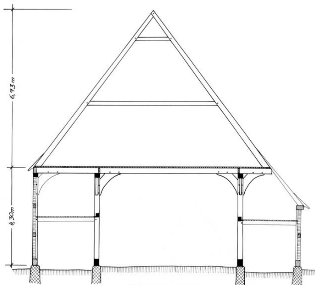
QUERSCHNITT A-B - REKONSTRUKTION -
