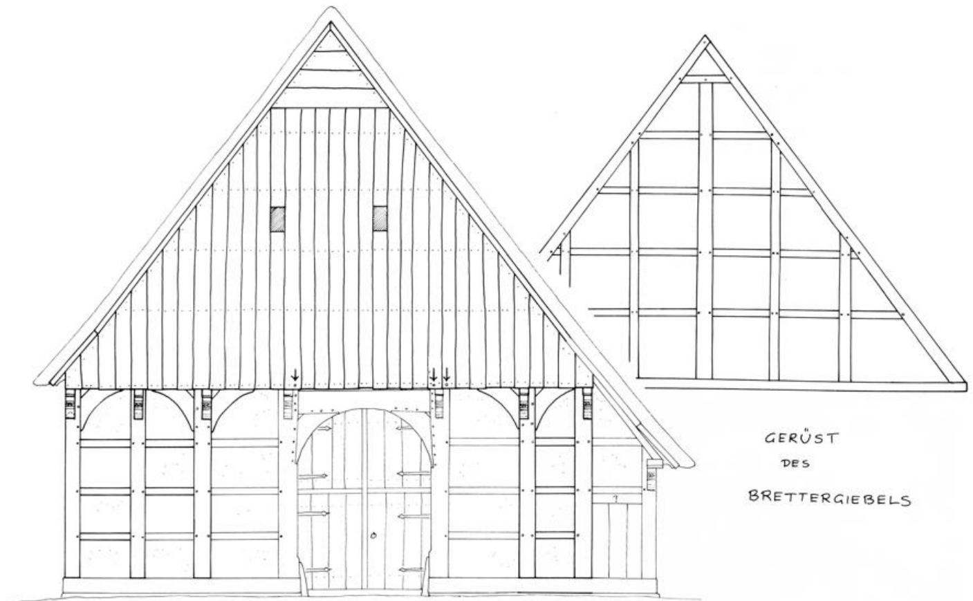
SÜD-GIEBEL - REKONSTRUKTION -
