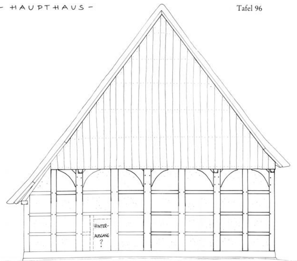
NORD - GIEBEL - REKONSTRUKTION DES URSPRÜNGLICHEN ZUSTANDES -
