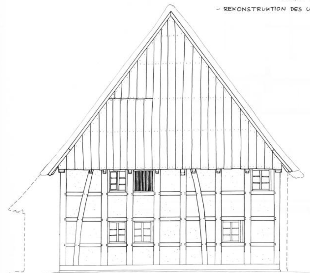
NORDGIEBEL DES KAMMERFACH - ANBAUS (MITTE 19. JAHRHUNDERT) - REKONSTRUKTION -
