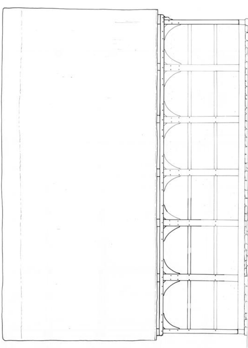
WEST - ANSICHT - REKONSTRUKTION -
