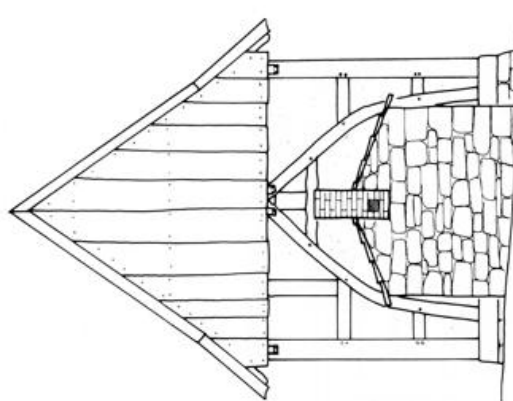
NORD-GIEBEL - ZUSTAND 1850 -
