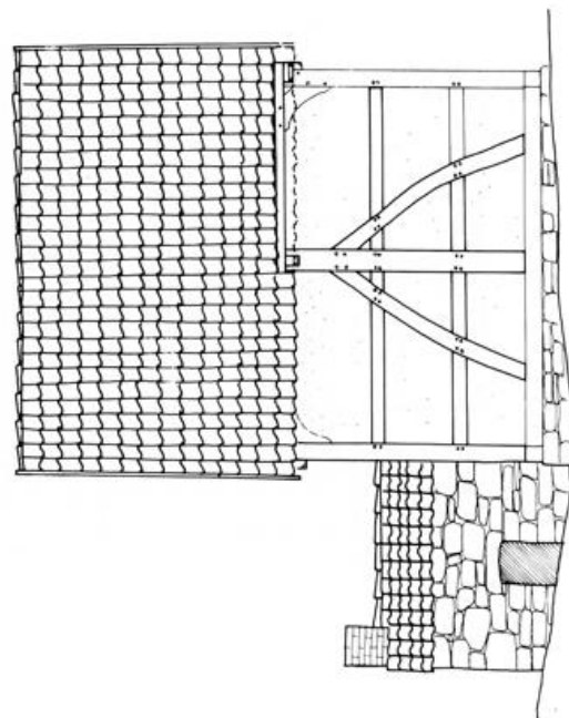
WEST-ANSICHT - ZUSTAND 1850 -
