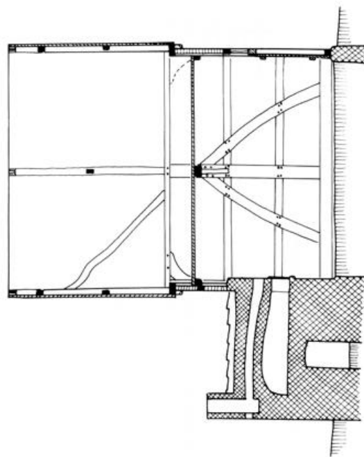
LÄNGENSCHNITT - ZUSTAND 1850 -
