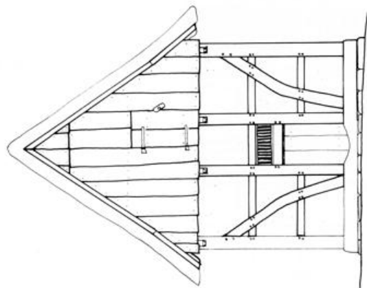
SÜD-GIEBEL - REKONSTRUKTION -
