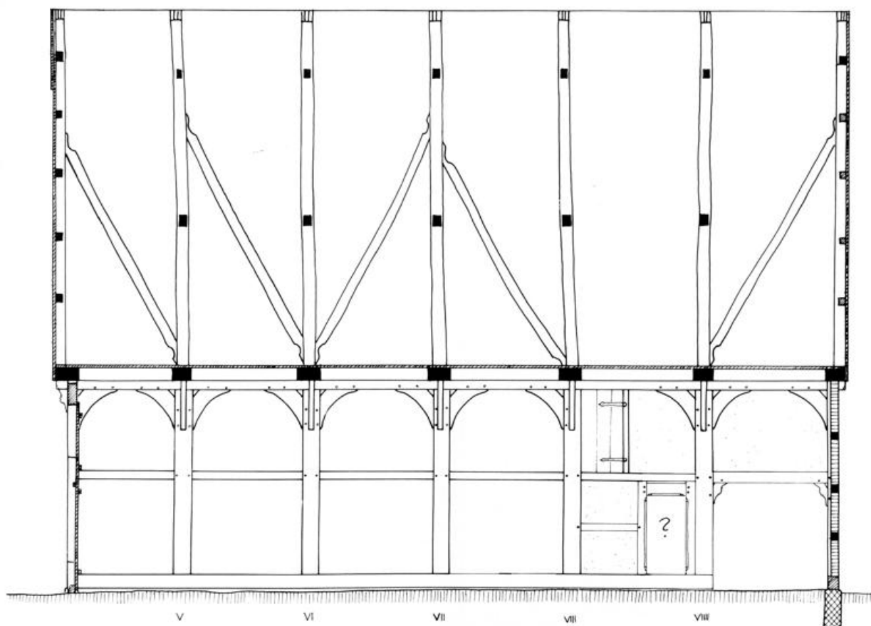
LÄNGENSCHNITT C-D - REKONSTRUKTION -
