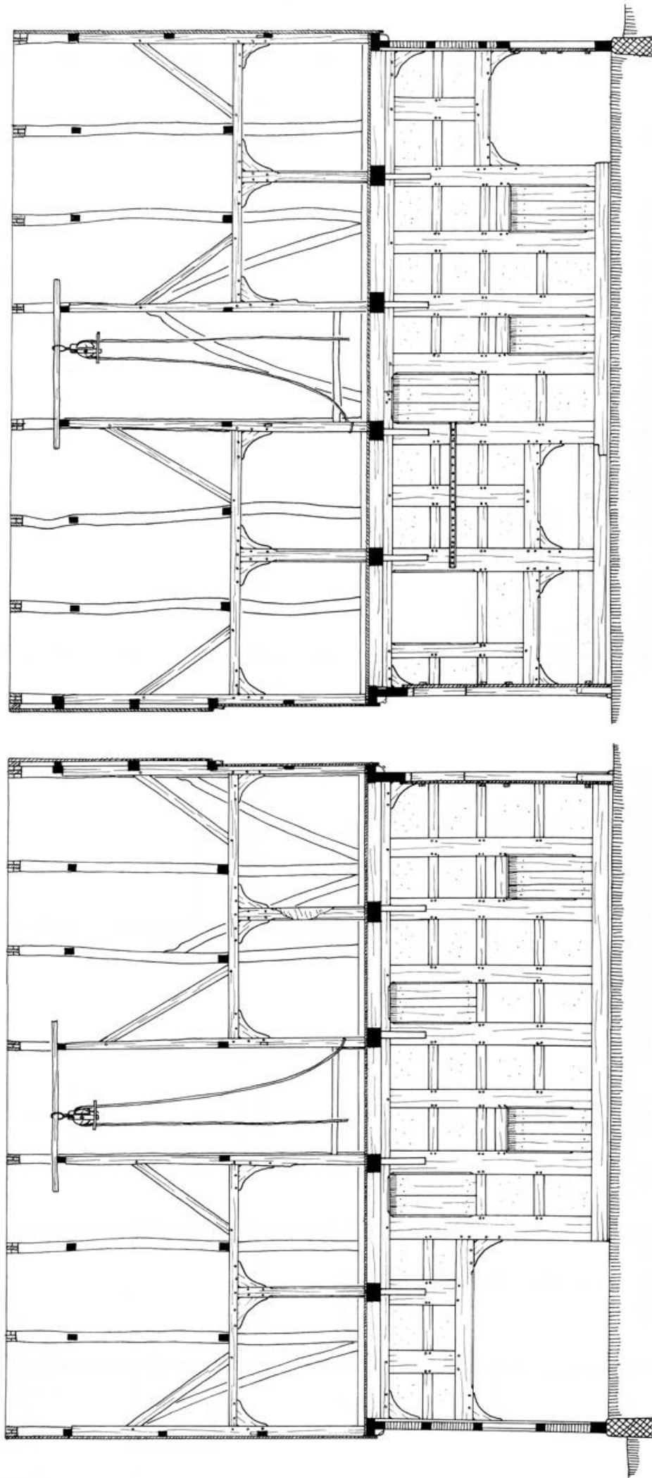
LÄNGENSCHNITT C-D
