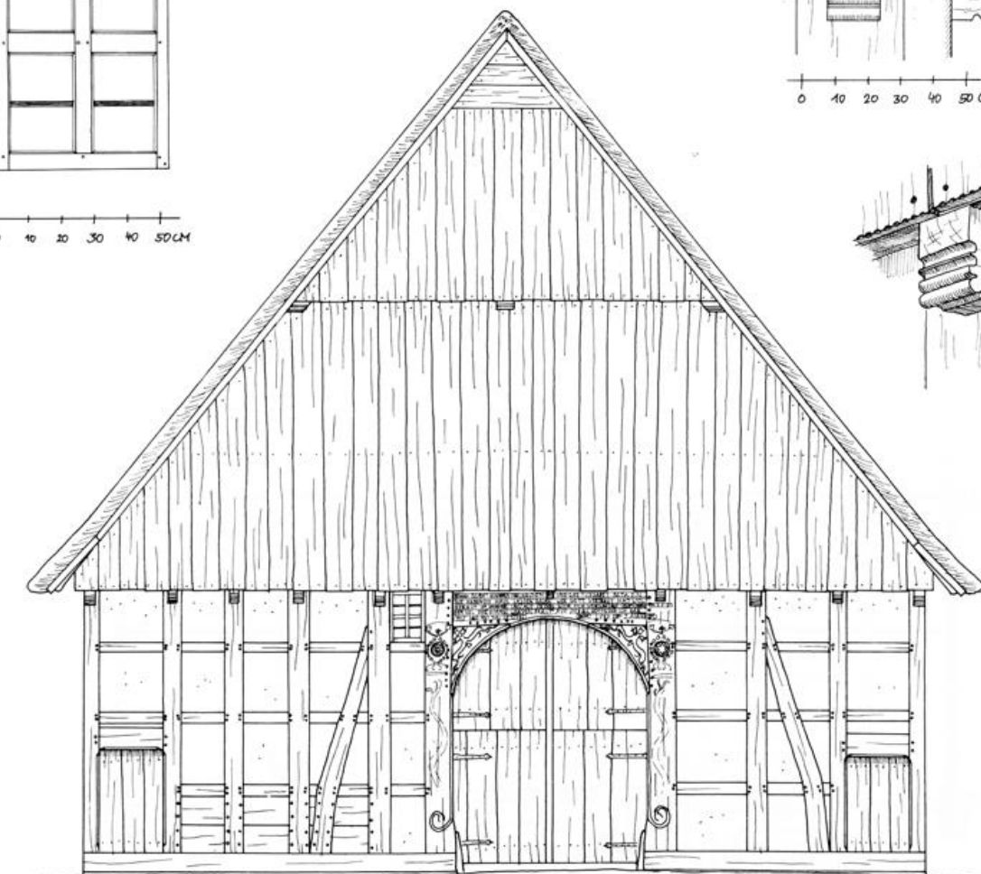
SÜD-ANSICHT -REKONSTRUKTION-
