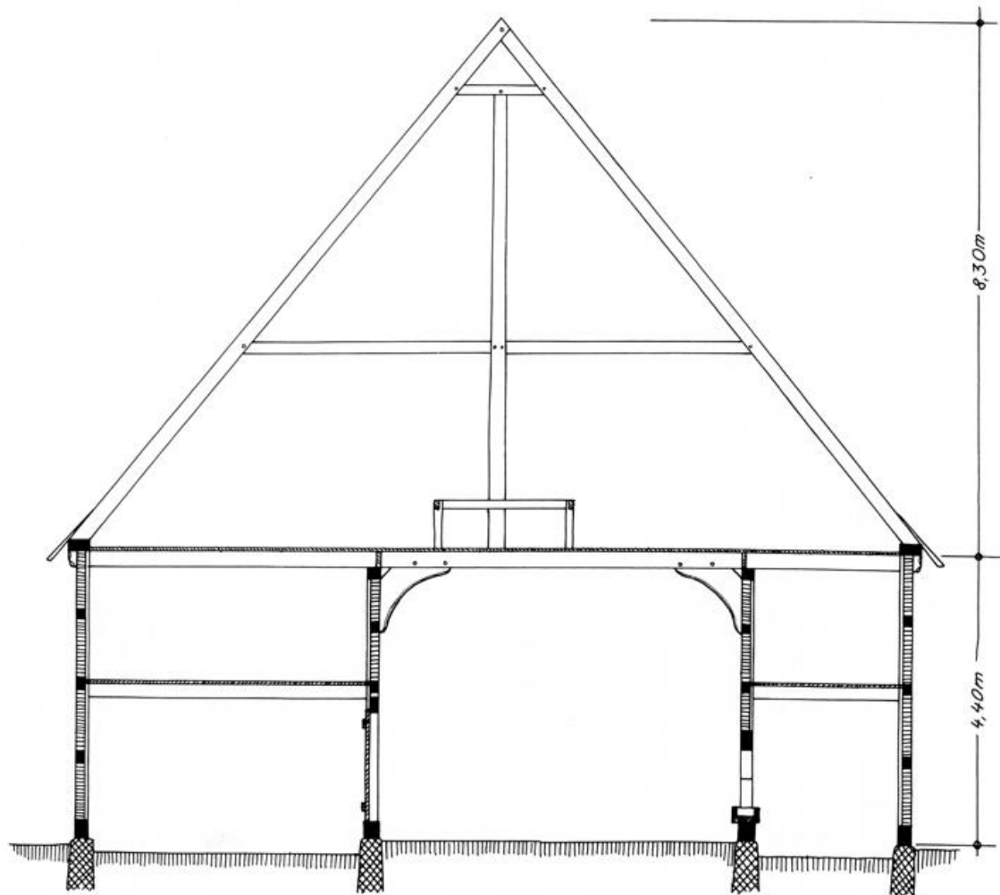
QUERSCHNITT E-F - REKONSTRUKTION -
