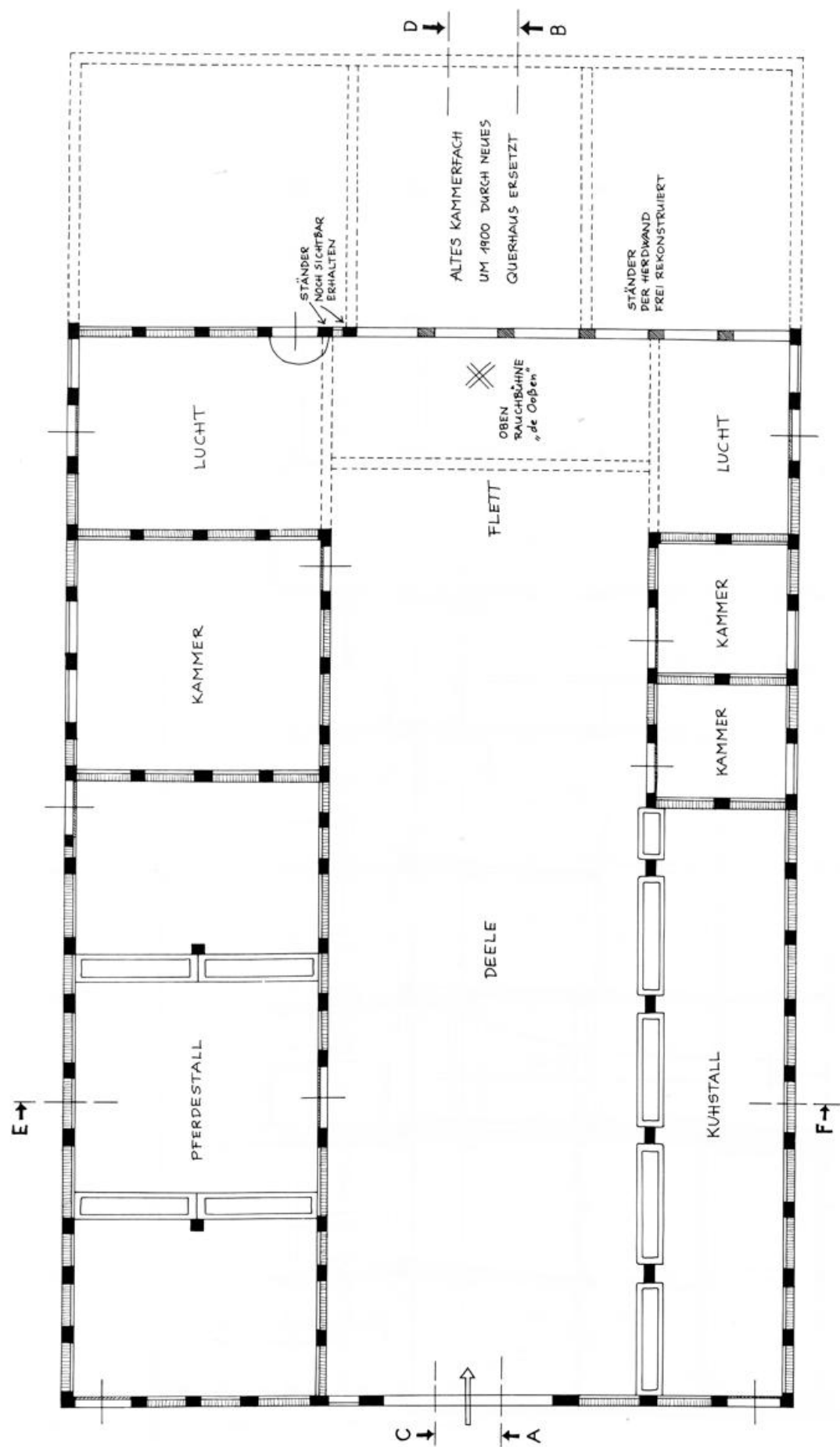
GRUNDRISS - REKONSTRUKTION -
