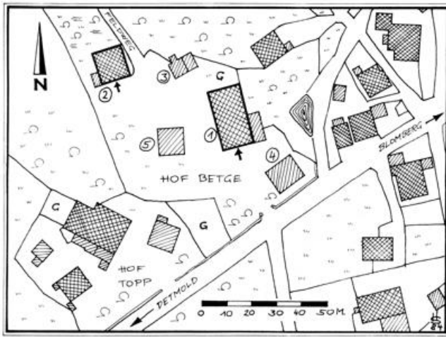
Abb. 55: Hof Betge in Vahlhausen. Lageplan nach Urkataster von 1880: (1) Haupthaus, 1743; (2) Leibzucht, 1686; (3) Backhaus; (4) Scheune, Pferdehaus?; (5) Scheune.
