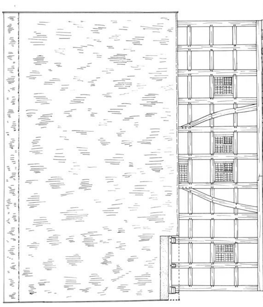
WEST-ANSICHT - REKONSTRUKTION -
