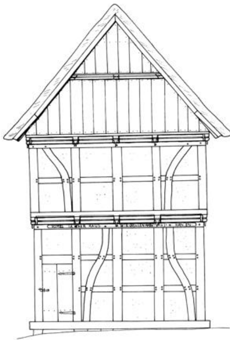
WEST - ANSICHT
