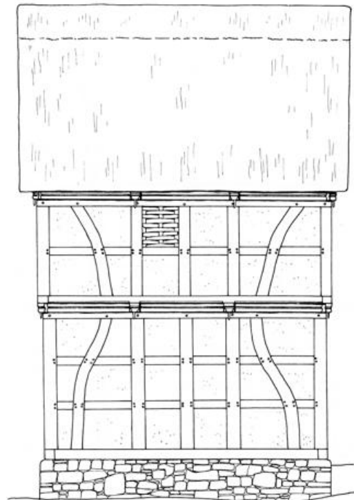
NORD - ANSICHT
