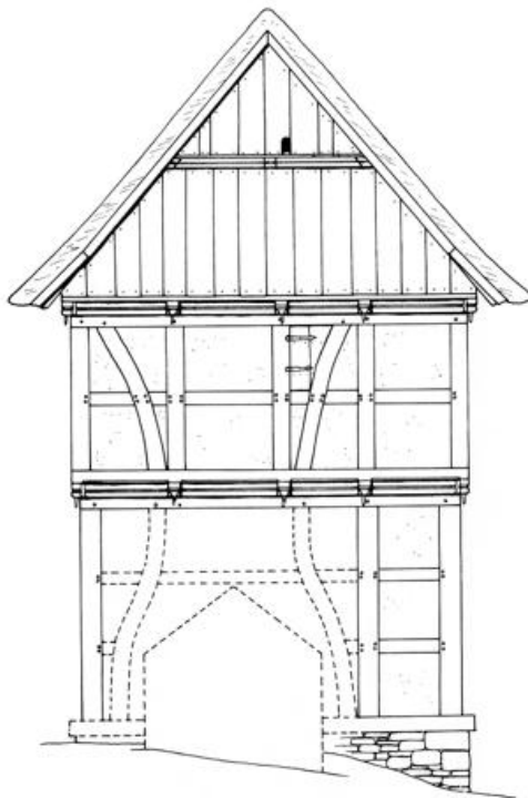
OST - ANSICHT
