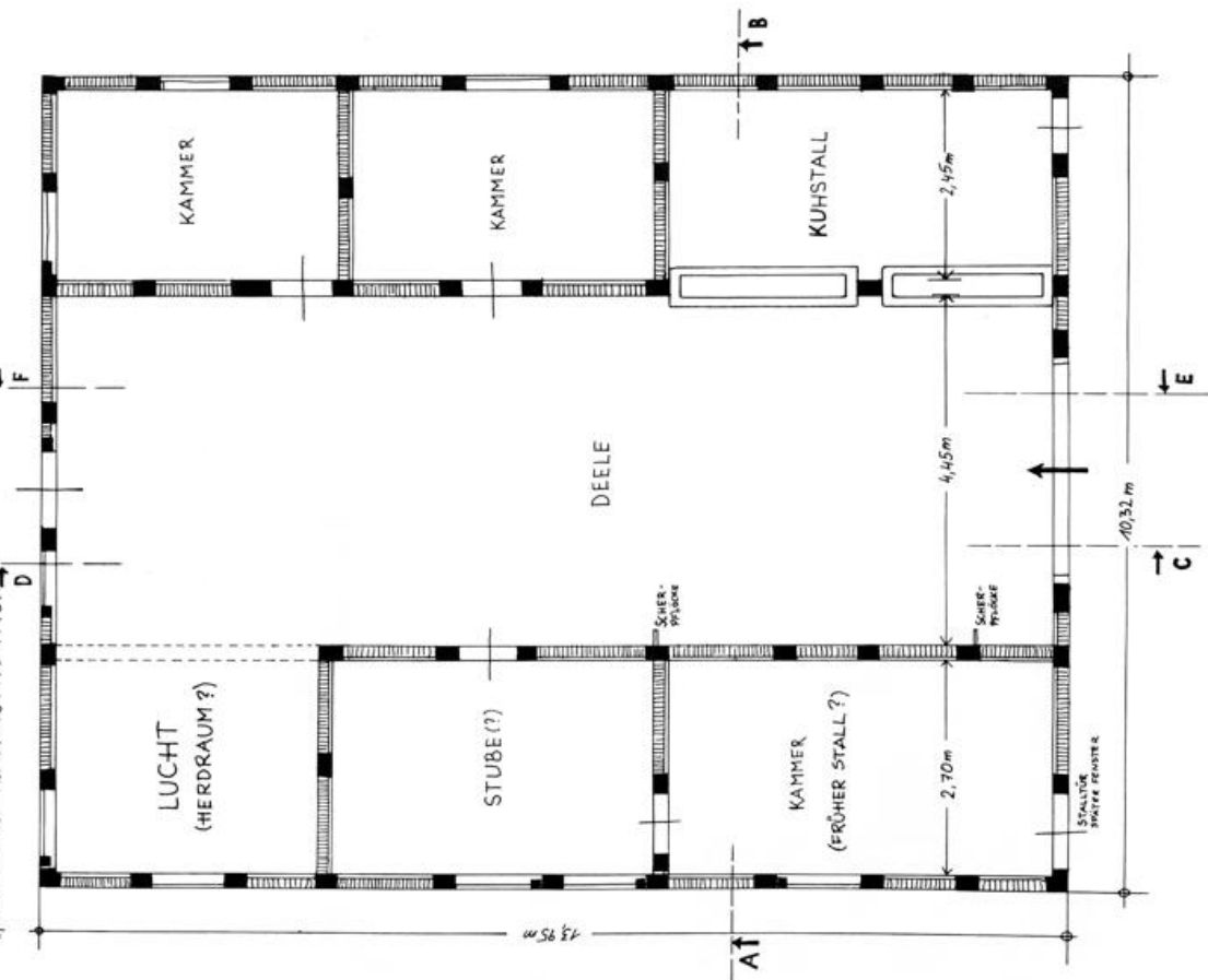
GRUNDRISS - REKONSTRUKTION
