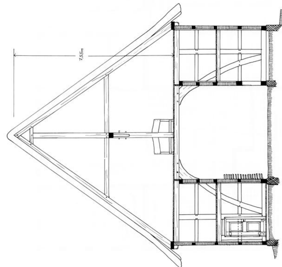
QUERSCHNITT A-B
