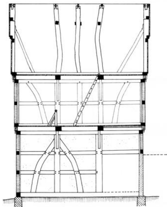
LÄNGENSCHNITT A-B
