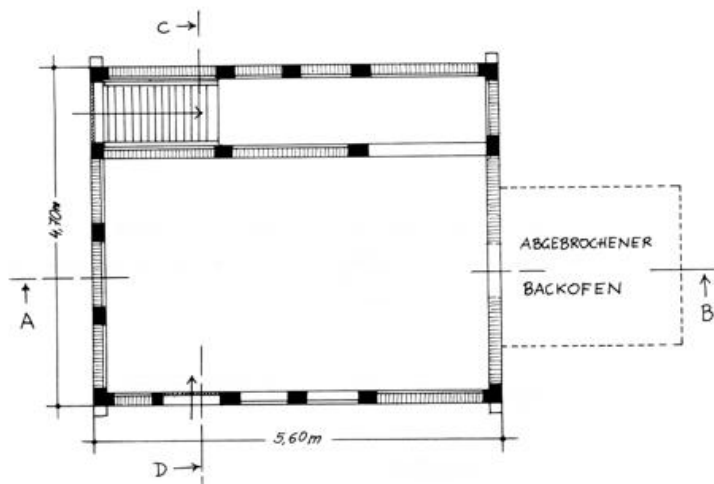
GRUNDRISS
