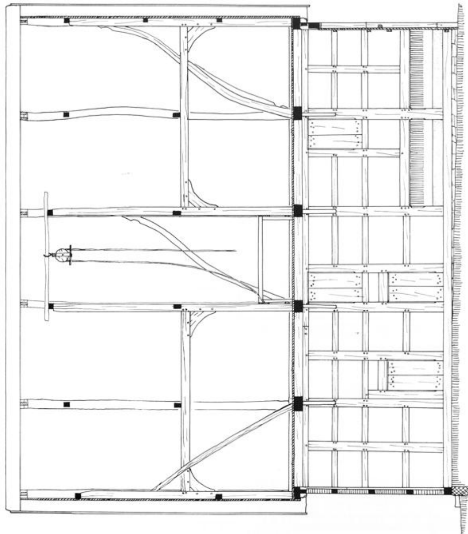
LÄNGENSCHNITT C-D
