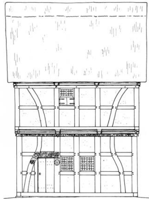
SÜD - ANSICHT
