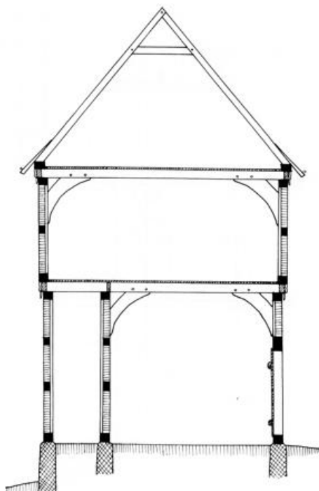
QUERSCHNITT C-D
